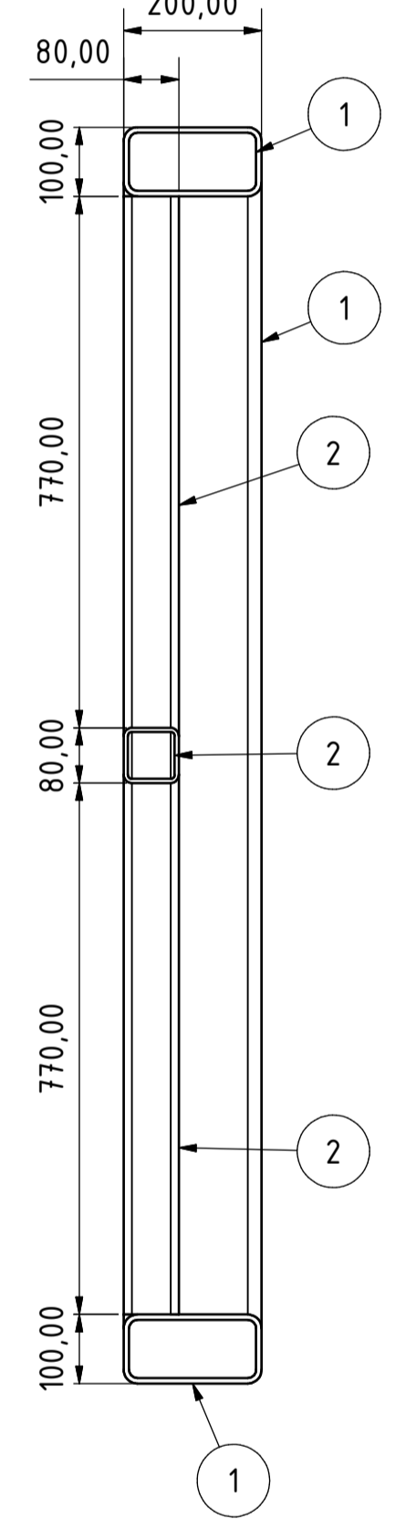
D-D ( 1 : 10 )
