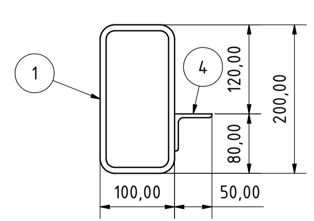
A-A ( 1 : 5 )
